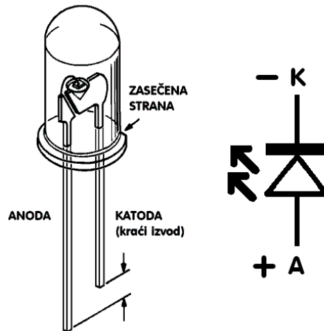
Izgled i polaritet LE diode
