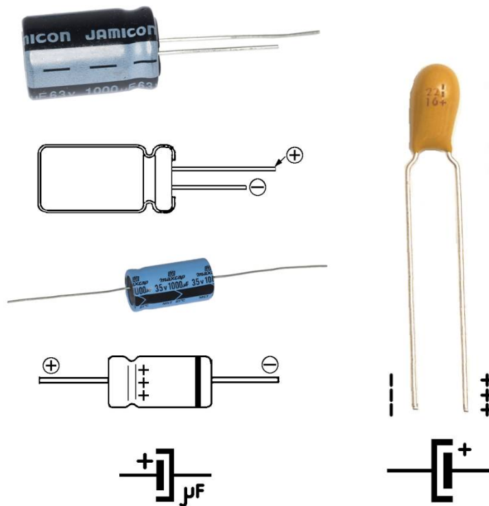
Izgled i polaritet elektrolitskih, odnosno tantal kondenzatora
